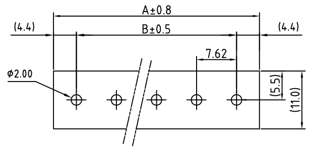
P.C.B LAYOUT
